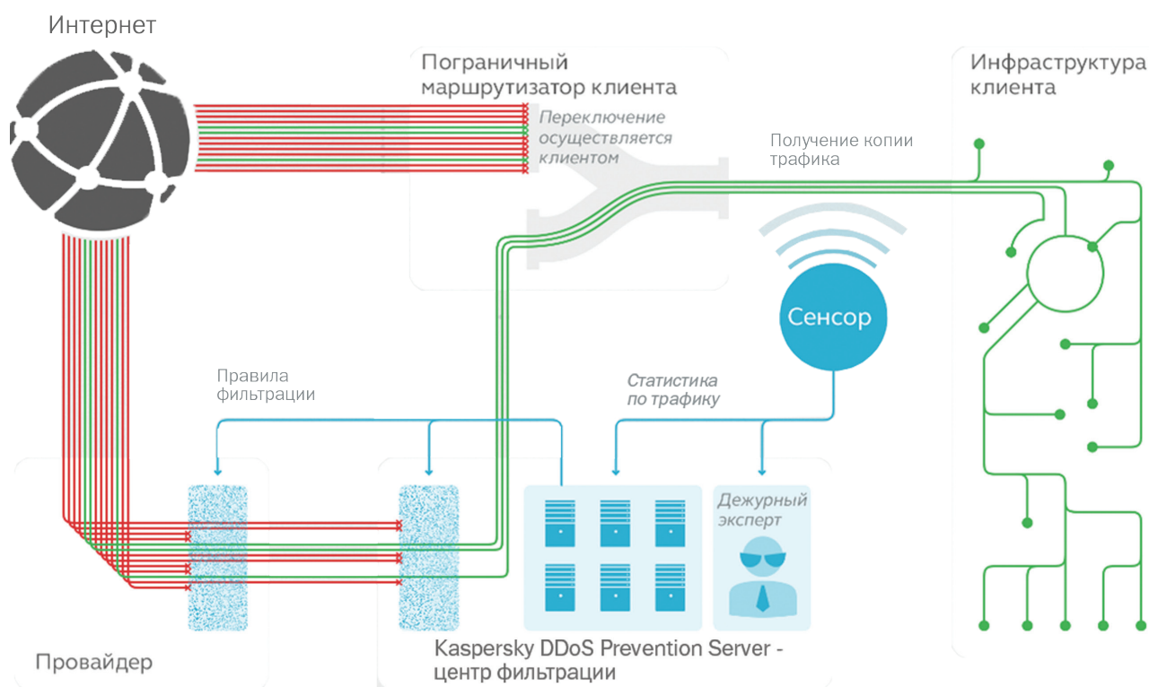
Рисунок 2. Схема работы Kaspersky DDoS Prevention
